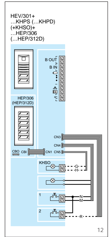
Fig.12 - Colore dei conduttori relativi ai cablaggi CN3-CN4-CN5.
